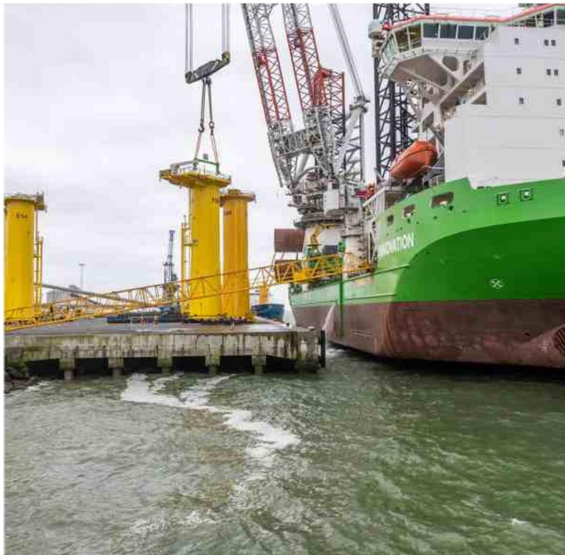
Au mois de mai 2021, les premières manutentions sur des embases d'éoliennes offshore sur les quais du Port Atlantique La Rochelle. Lequel entend maintenant se positionner sur la construction et la maintenance du parc prévu au large d'Oléron. ARCHIVES XAVIER LÉOTY / SO
